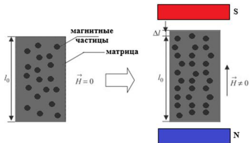
Рис. 1. Схема магнитореологического эффекта
